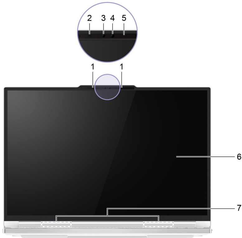
Abbildung 1. Legion 7 16IAX10—Vorderansicht
