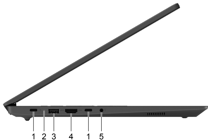
Abbildung 5. 15-Zoll-Modelle—Ansicht von links
