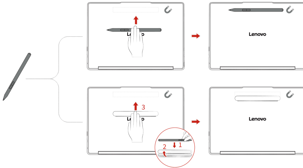
Abbildung 15. Stiftbefestigung an der oberen Abdeckung des PCs
